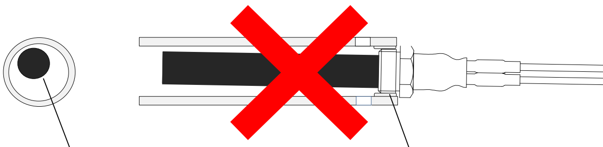
Heizelement ist in Kontakt mit dem Schutzrohr
